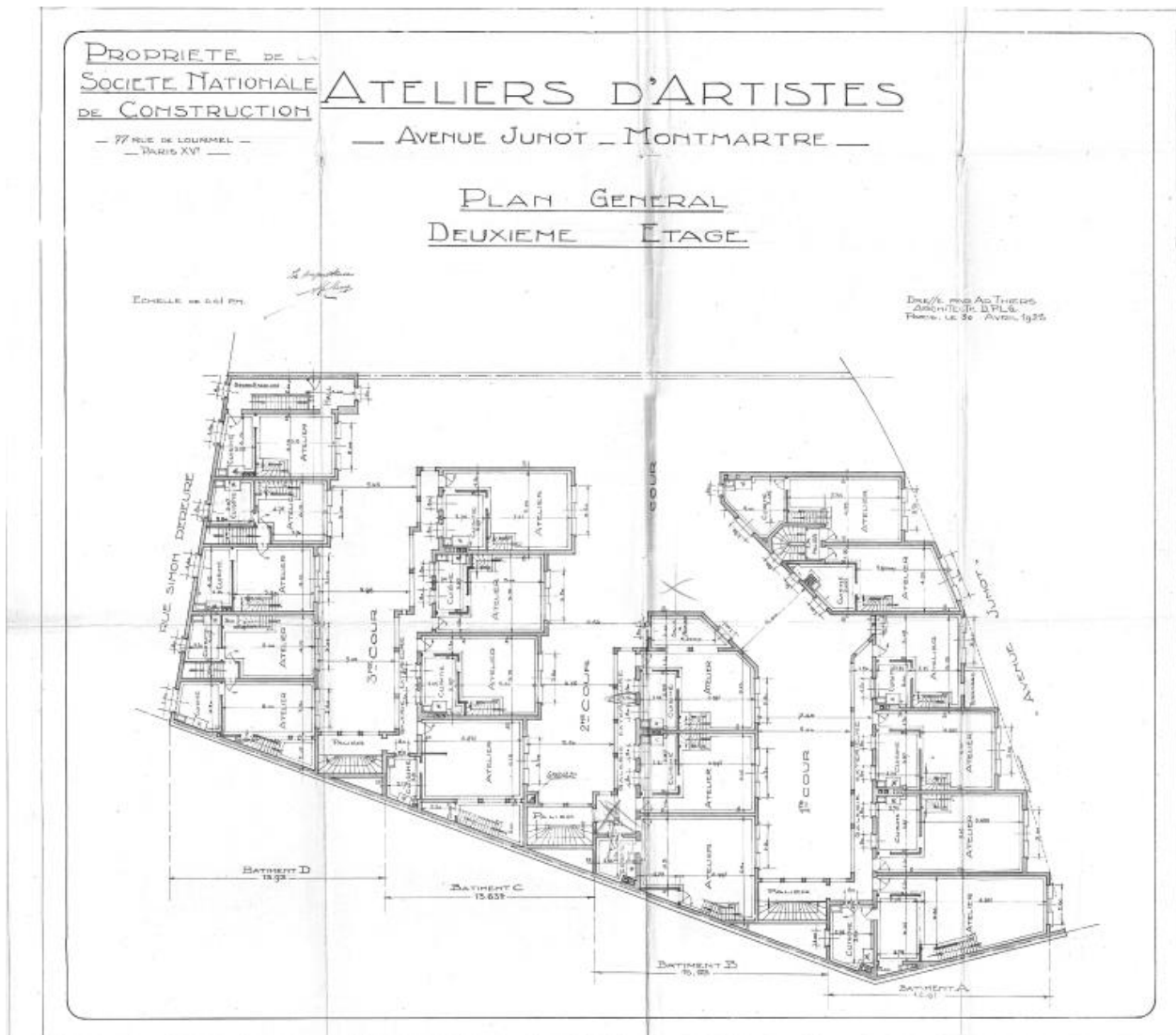
Plan général du deuxième étage
