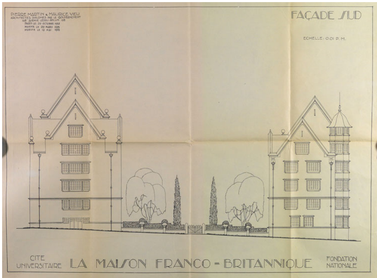
Façade sud, par Pierre Martin et Maurice Vieu ; 20 octobre 1932, modifié les 20 mars et 10 mai 1933. Plan. Archives nationales, AJ 16/7041.
