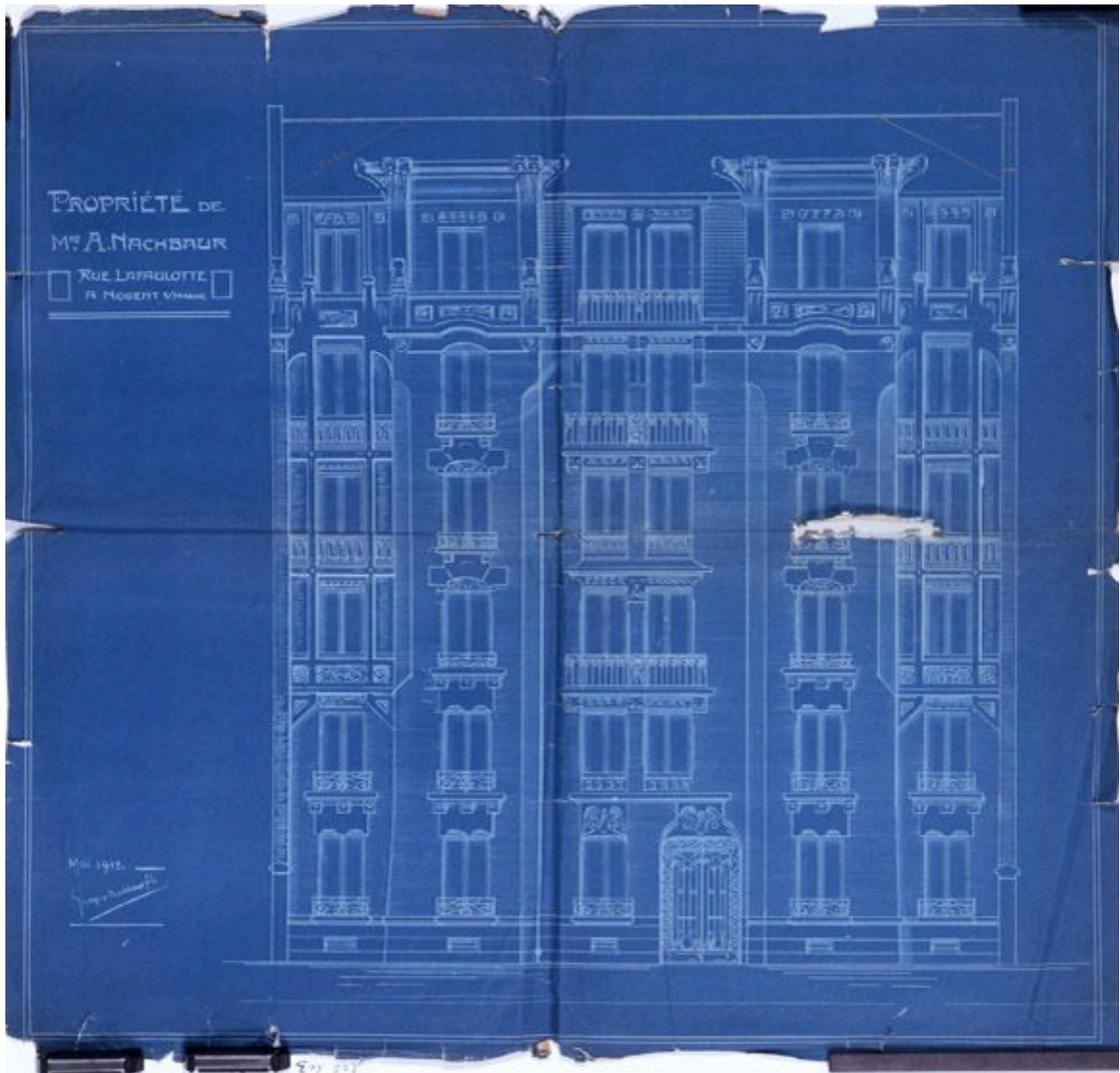
Plan de demande d'autorisation de construire pour Mr Nachbaur. Elévation. Signé et daté Nachbaur mai 1912. (AM Nogent-sur-Marne. 1 02 103)
