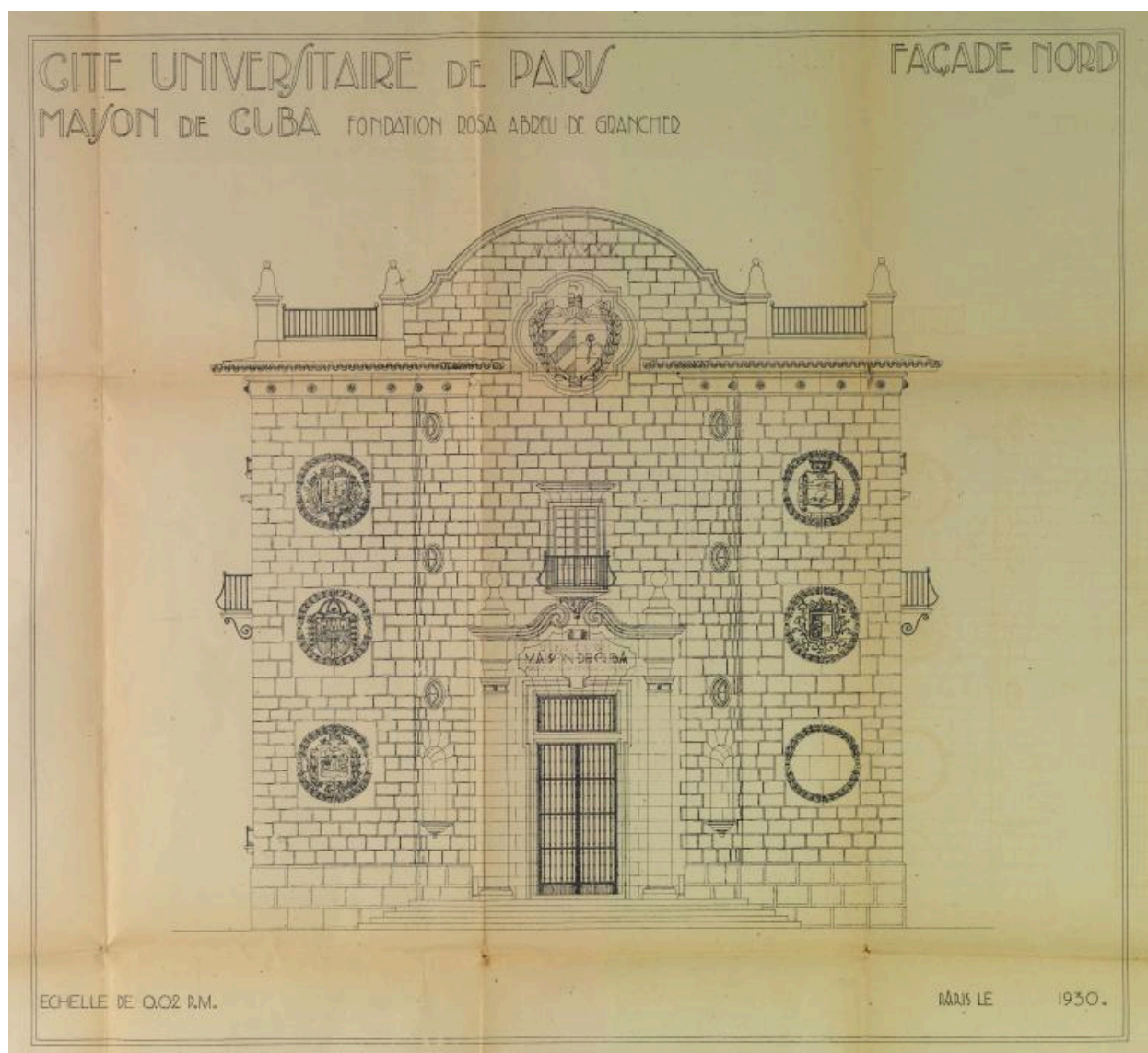
Élévation nord ; A. Laprade, architecte, 1930. Plan. Archives nationales, 20090013/318.
