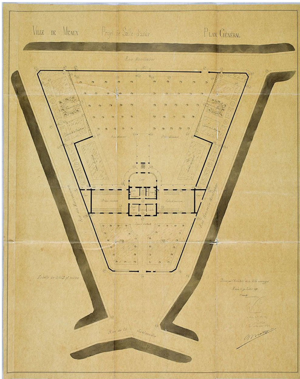
Projet de la salle d'asile rue Monthabor, plan général. Calque. (AD Seine-et-Marne. 4 Op 284/8)
