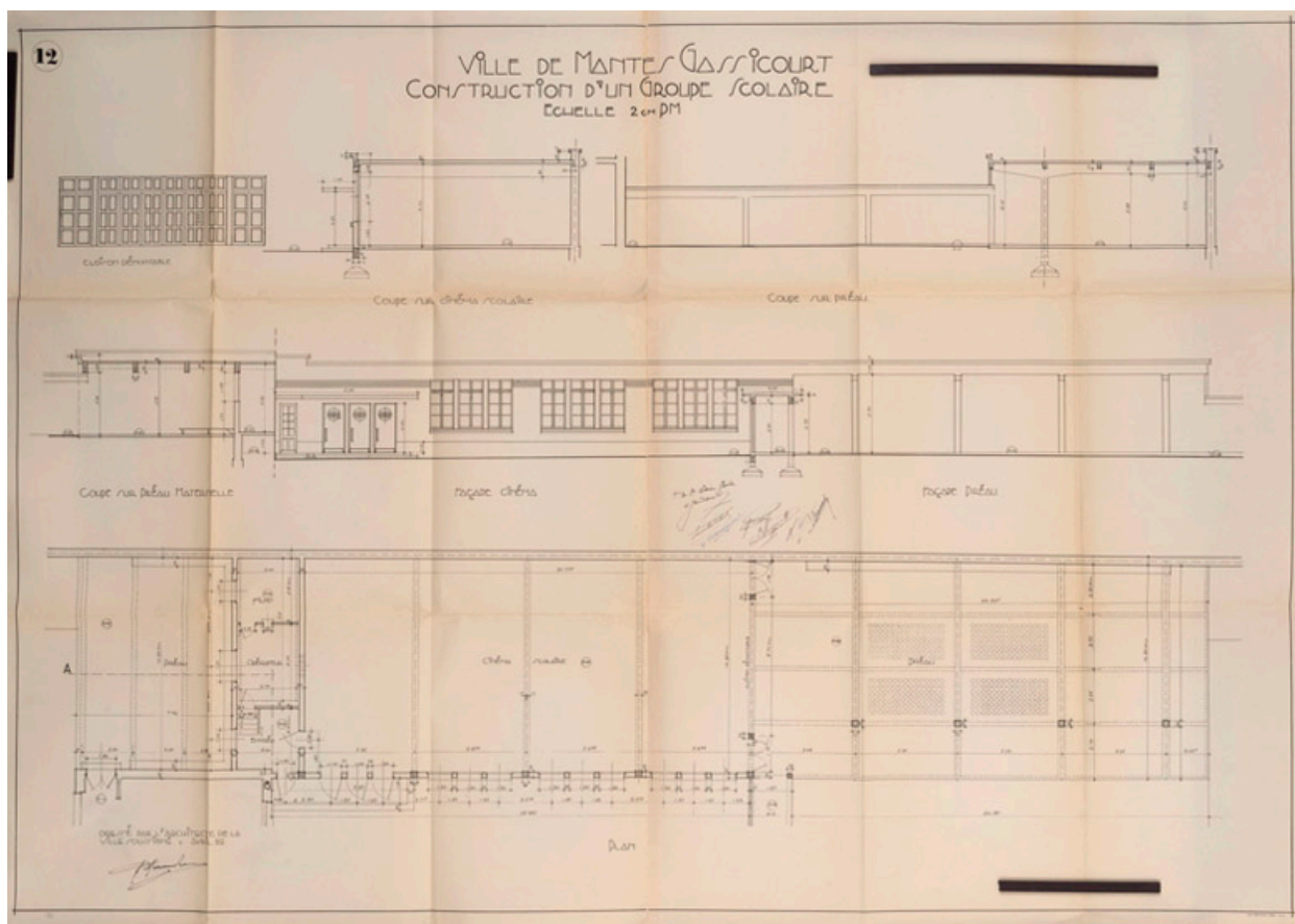
Plan et façades du cinéma scolaire. Marabout. 1932 (AM Mantes-la-Jolie 5 M 15 (2))
