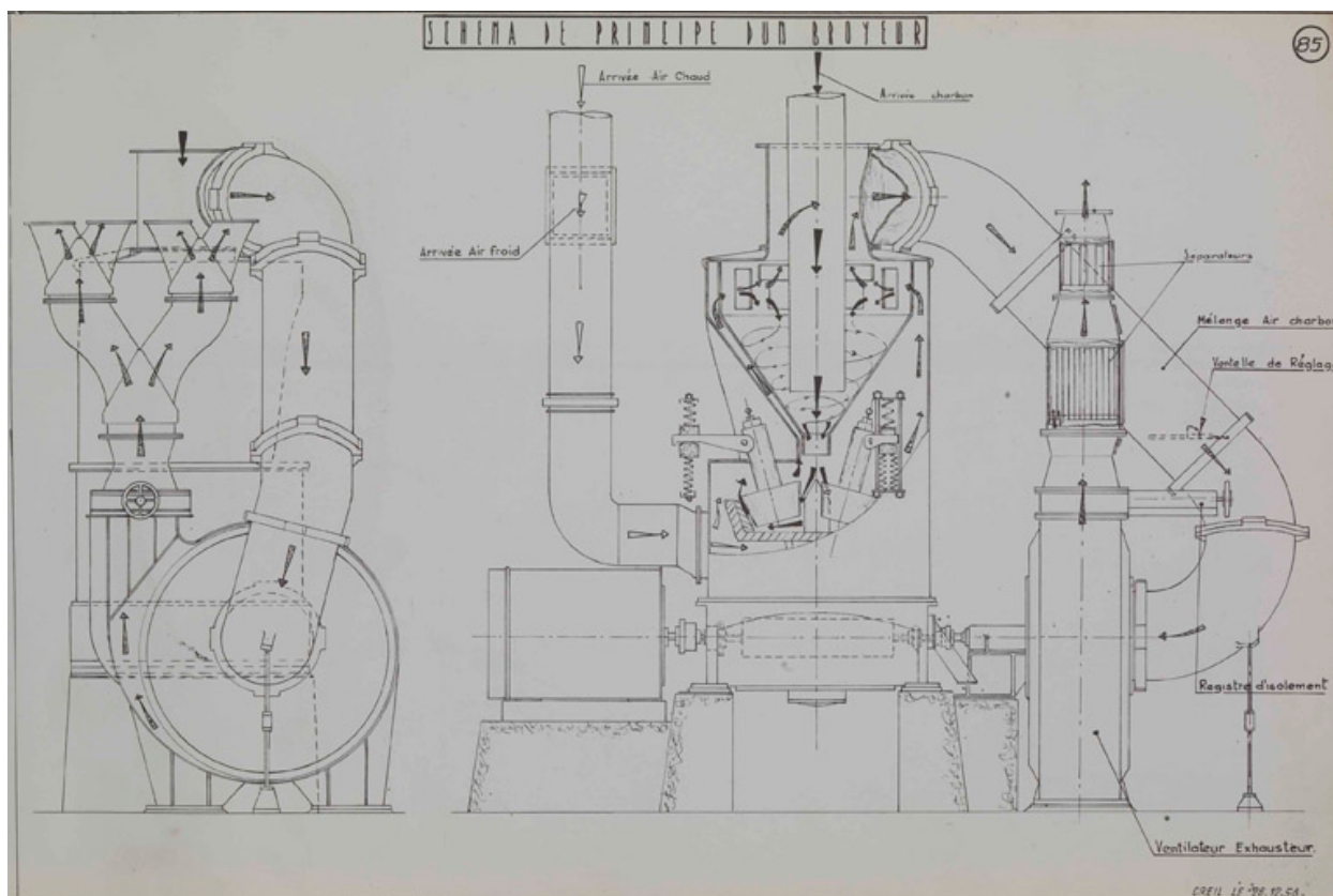
Schema de principe du broyeur.
