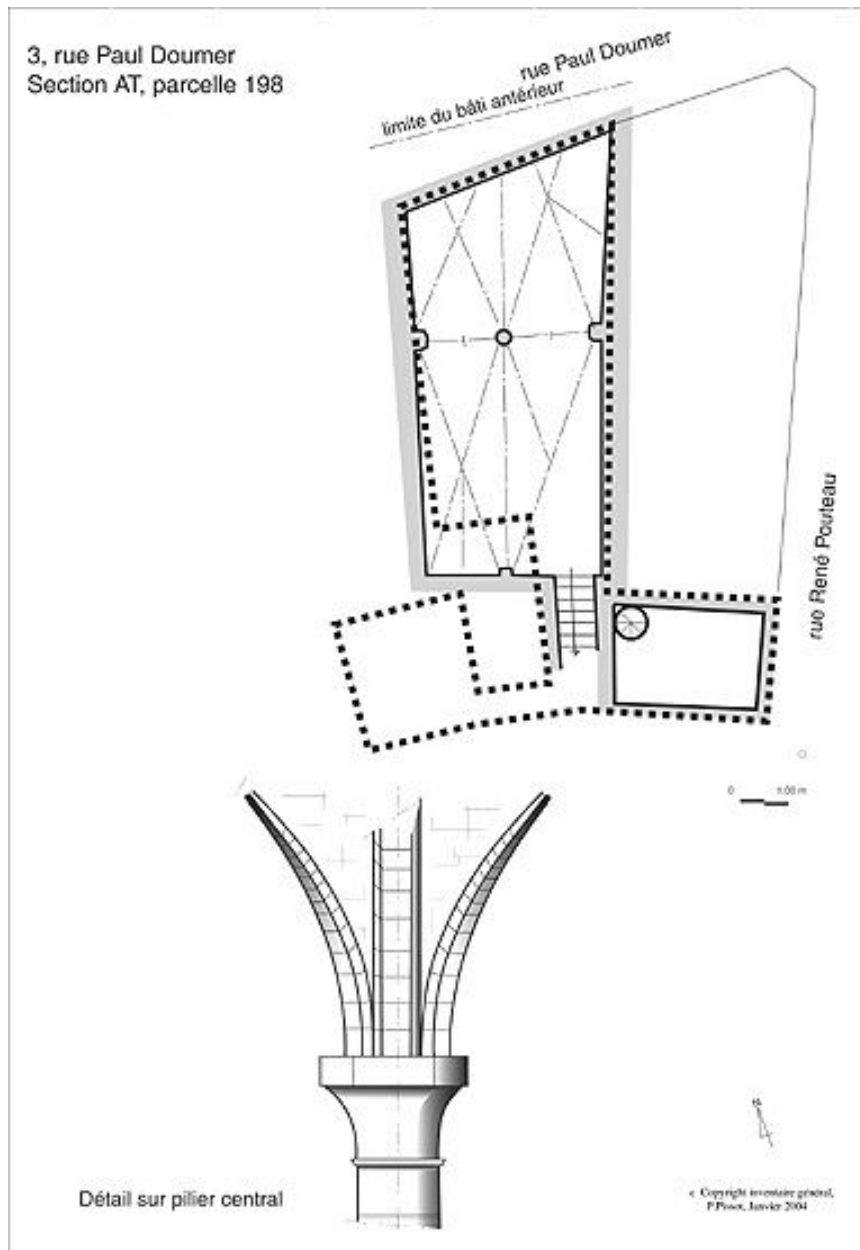
Plan de la cave médiévale et détail du pilier central.
