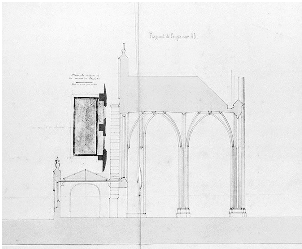
Ville de Melun. Eglise Saint-Aspais. Construction d'une nouvelle sacristie. Coupe sur l'église et la sacristie, plan du comble de la nouvelle sacristie. Papier aquarellé, 1863 (10 juin). (BM Melun. HH 31)
