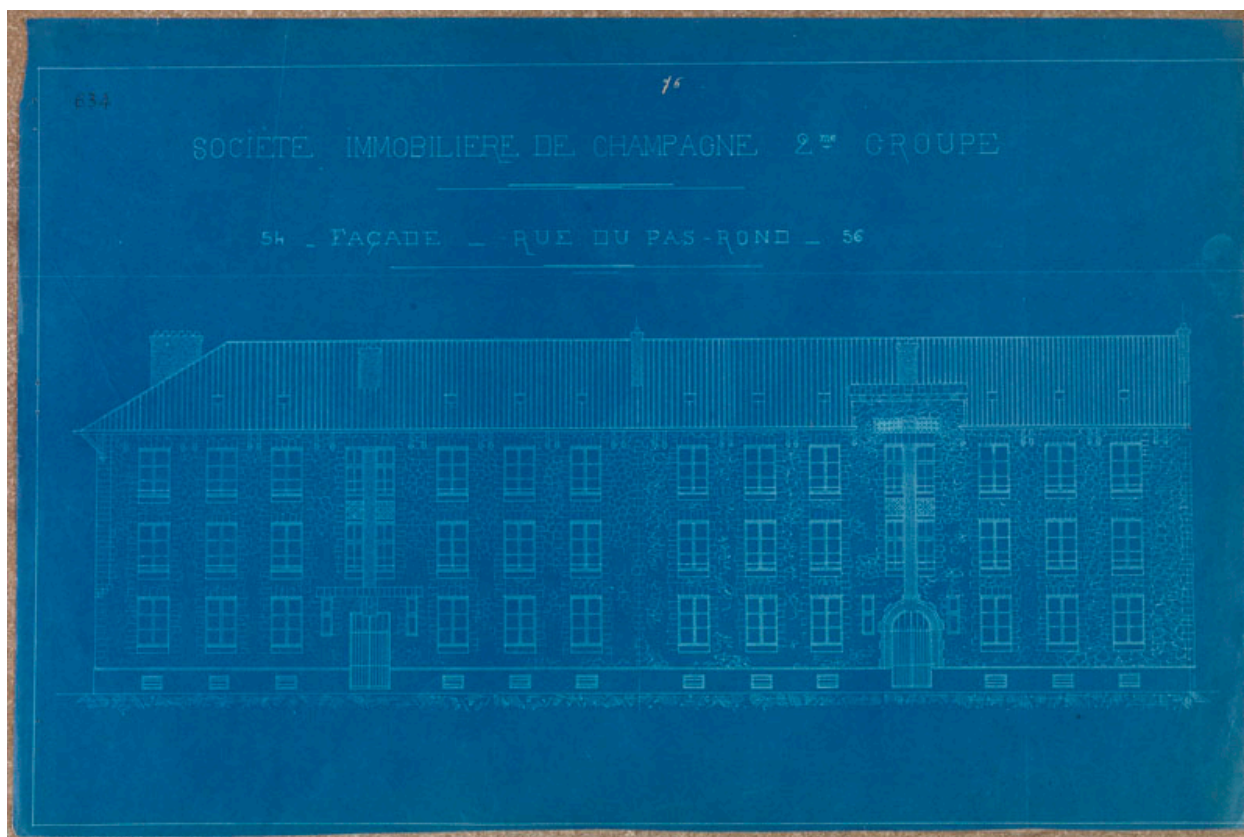
Plan. Société immobilière de Champagne. Façades. 2e groupe, 54/56 rue du Pas-Rond
