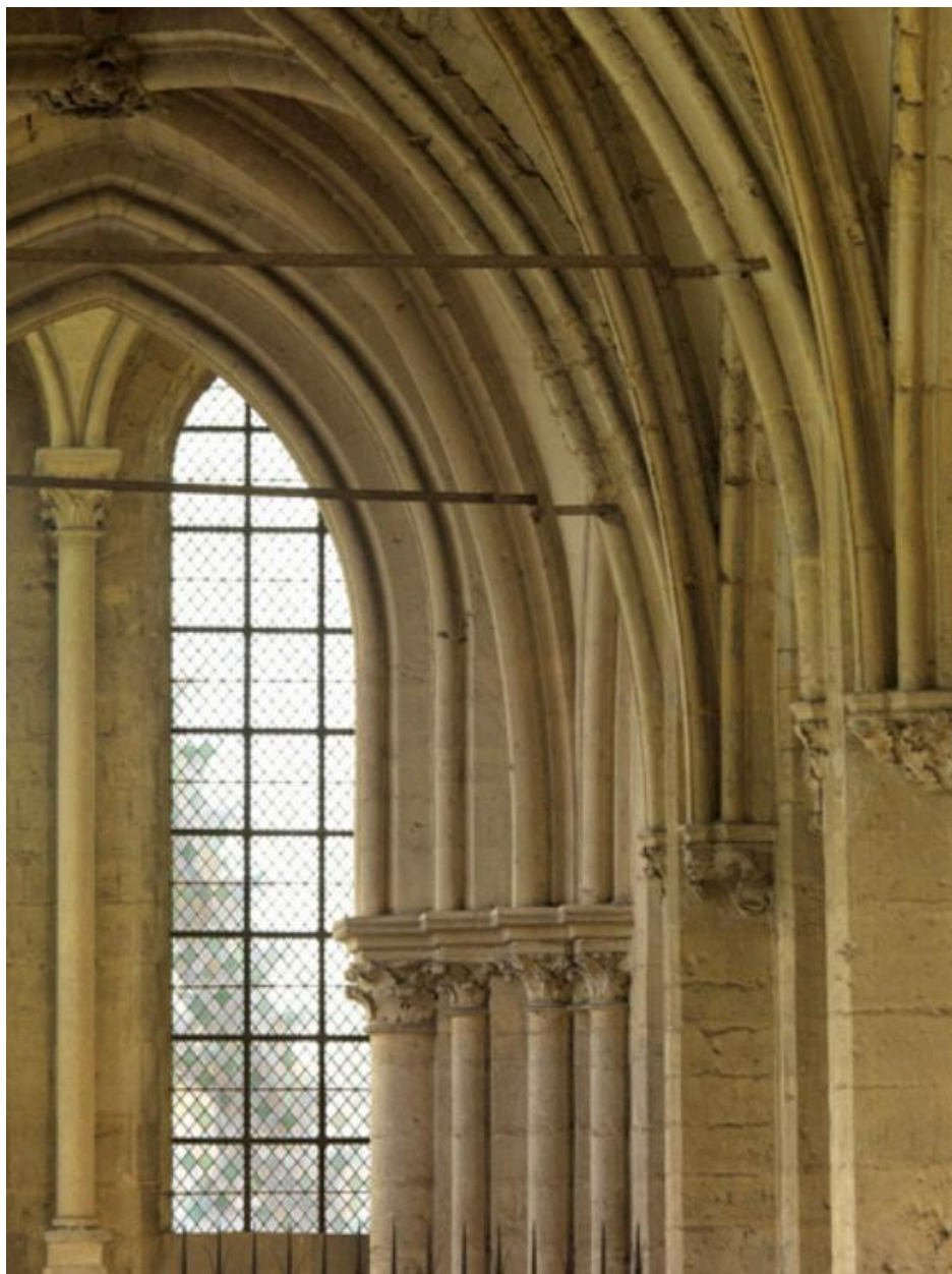
Tirant de fer maintenant les voûtes en place.
