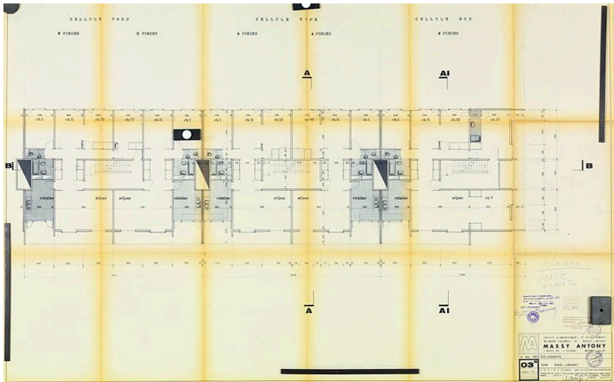
Plan d'étage courant. (AM Massy, 7 T 74)
