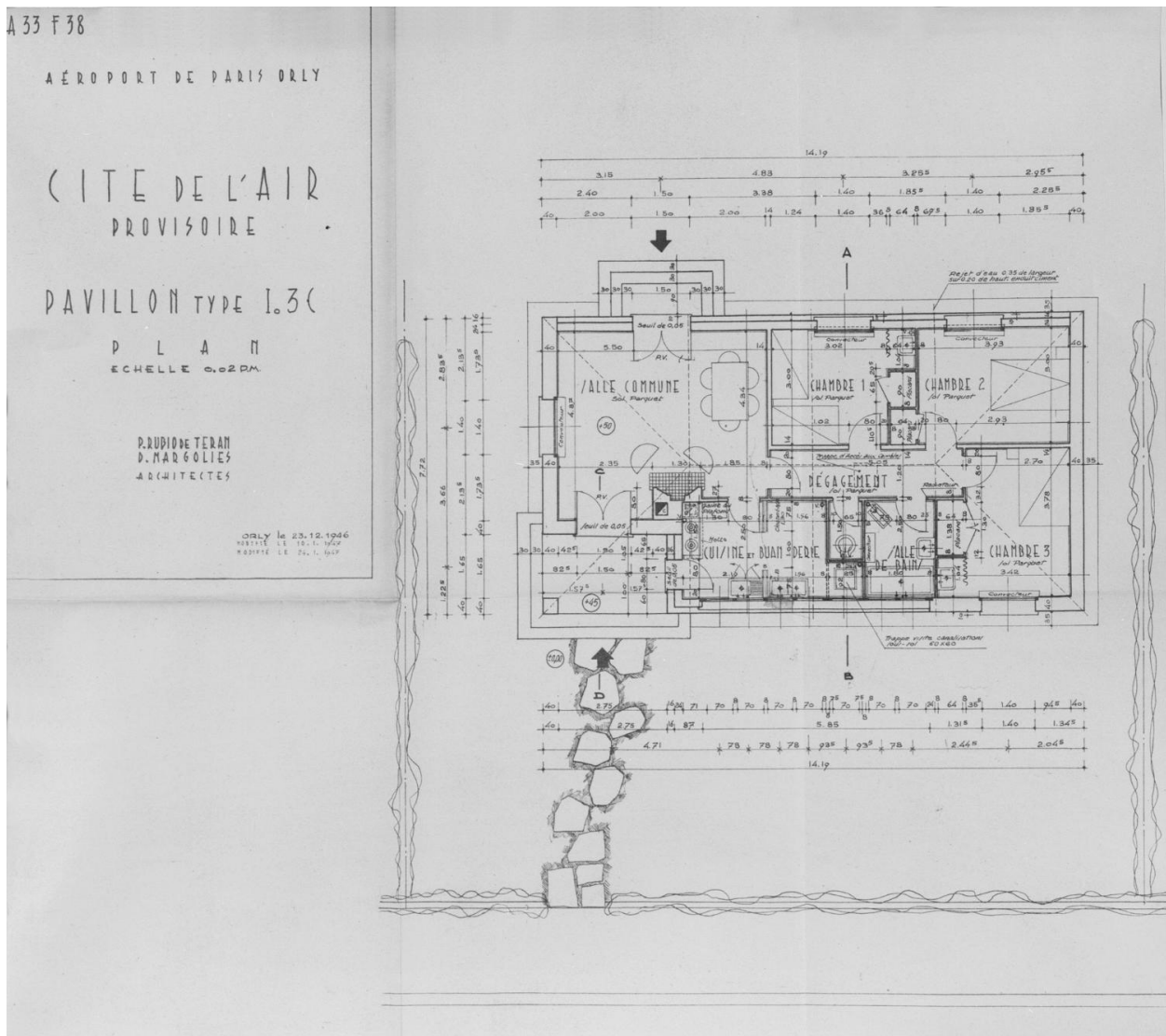
Plan d'un pavillon du type I 3 C, dressé par les architectes Rubio de Teran et Margolies, 23 décembre 1946 ; modifié en janvier 1947.
