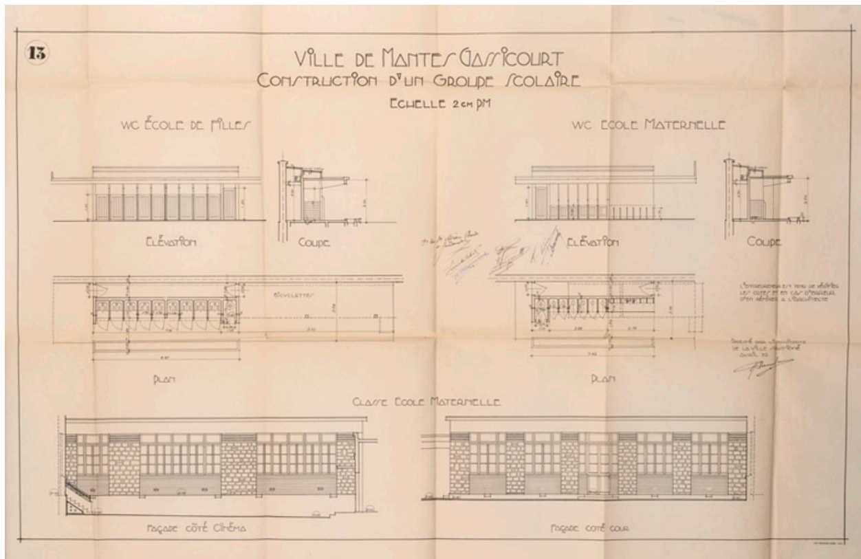
Plans et élévations des sanitaires. Marabout. 1932 (AM Mantes-la-Jolie 5 M 15 (2))
