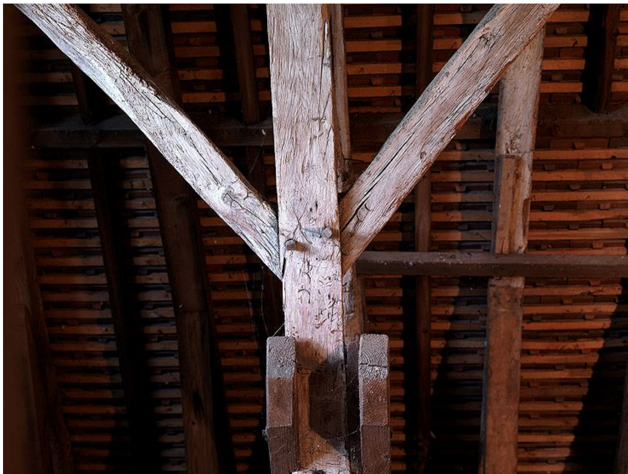
Détail des marques d'assemblage inscrites à la gouge sur la charpente du bras sud du transept, côté ouest (3e poteau en partant du sud).
