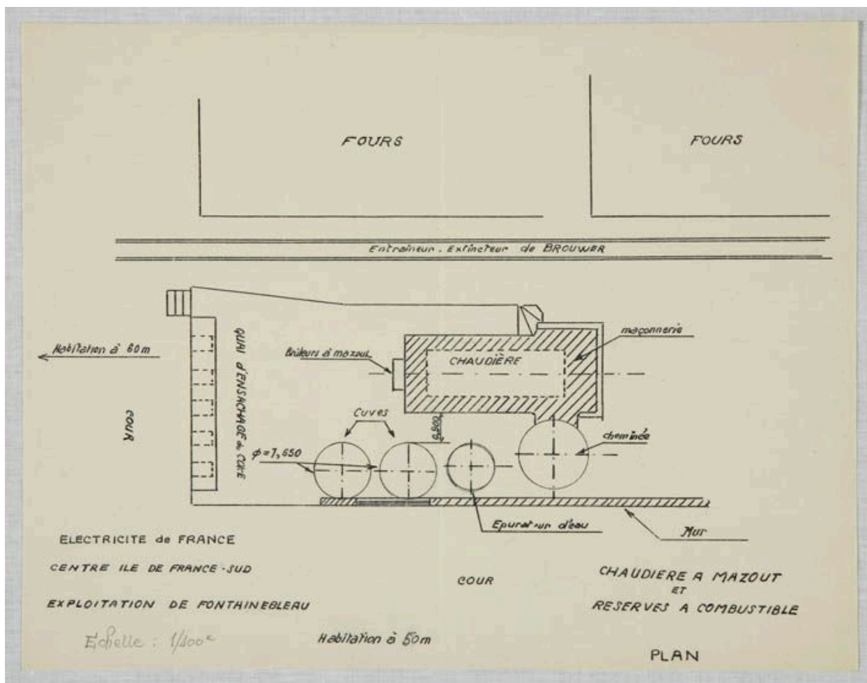
Plan de situation de la chaudière à mazout, 1949. (AD Seine-et-Marne, 5MP184)
