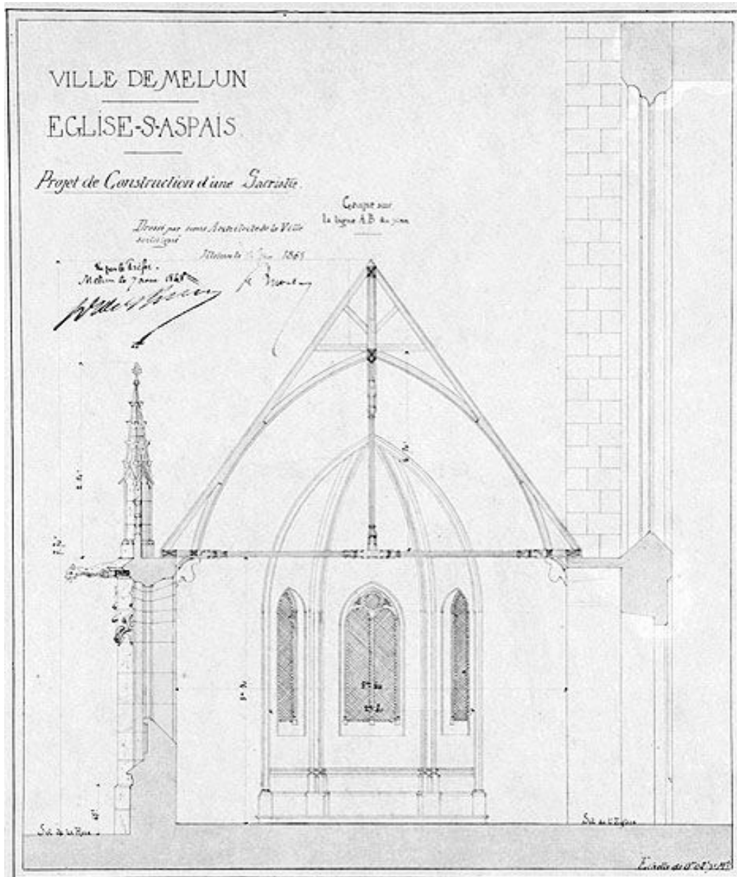
Ville de Melun. Eglise Saint-Aspais. Projet de construction d'une sacristie. Coupe transversale. Ech. 0.02 m.p.m. Calque aquarellé, 12 juin 1868. (BM Melun. HH 29)
