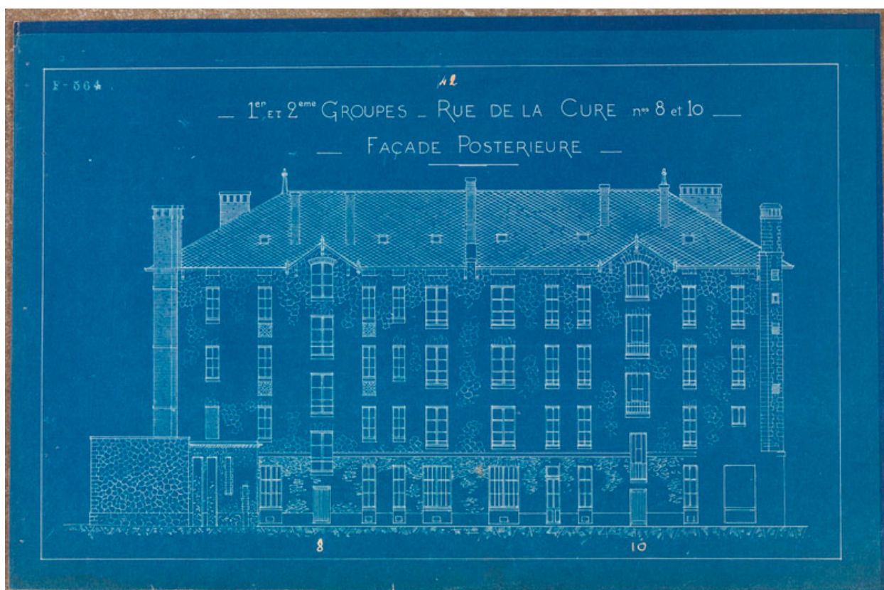
Plan. Société immobilière de Champagne. Façade postérieure. 1er et 2e groupes, 8 et 10 rue de la Cure.
