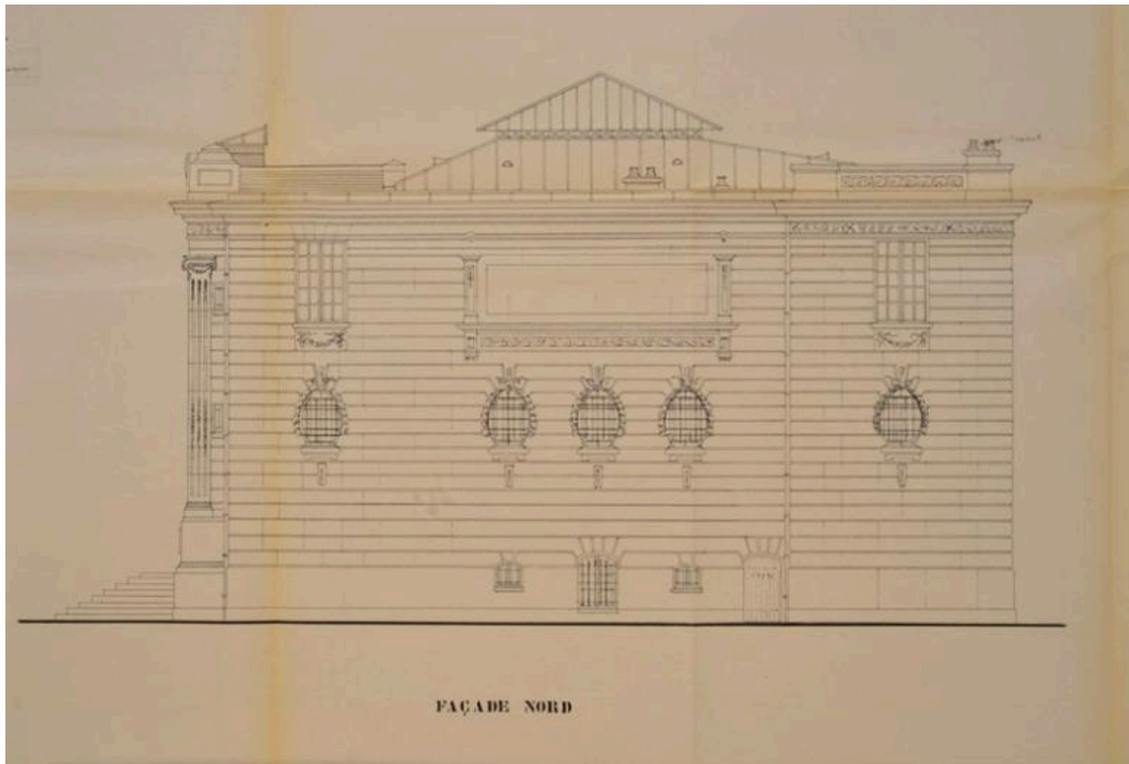
Relevé de la façade nord. Projet de restauration en 1981. Tirage. (AM Mantes-la-Jolie 53 W 123)
