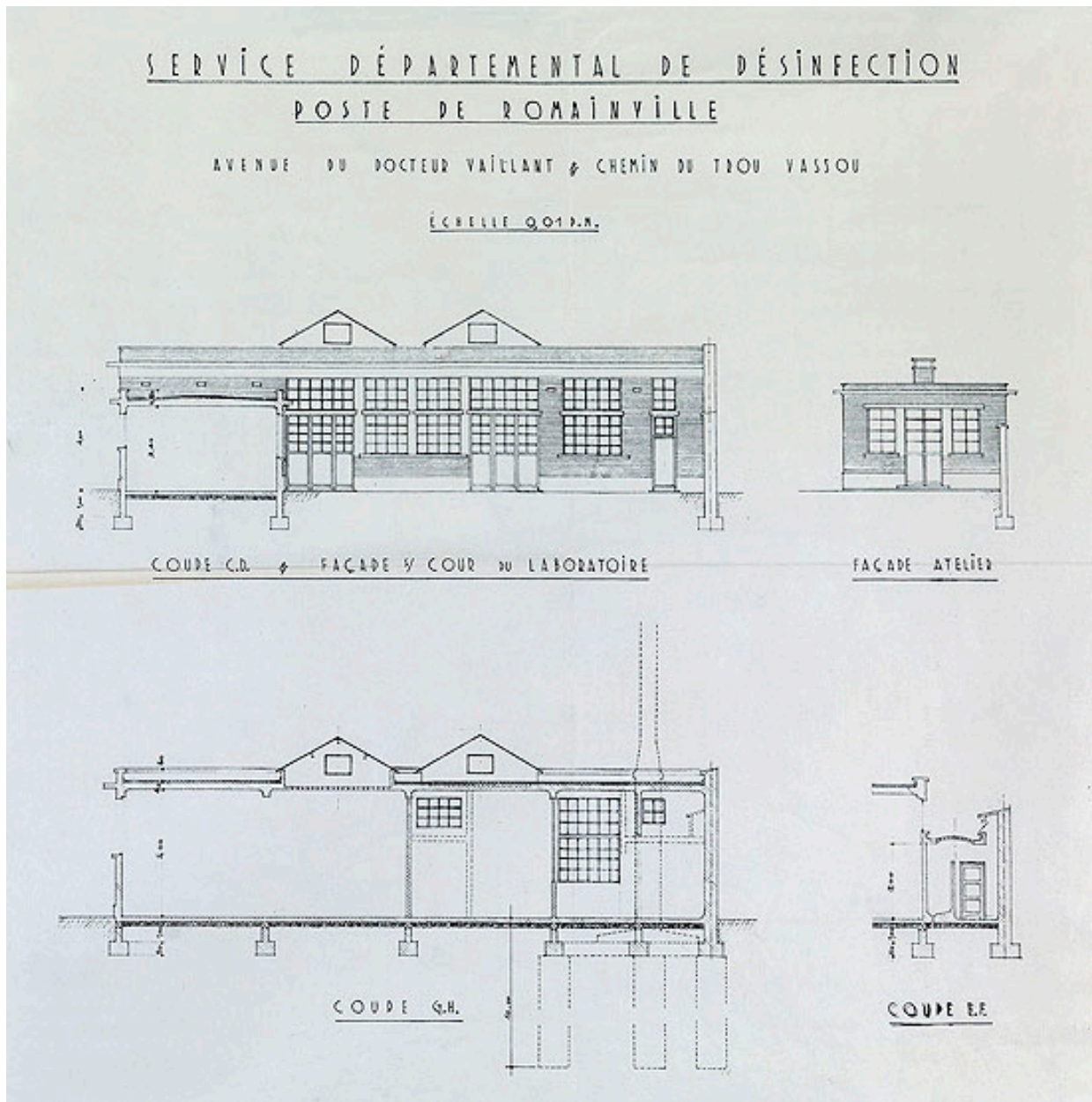
Coupes et façade sur cour du poste de désinfection de la préfecture de police, avenue du Docteur Vaillant et chemin du Trou Vassou. (AD Seine-Saint-Denis)
