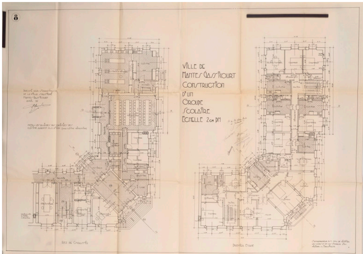
Plan du rez-de-chaussée et de l'étage du bâtiment d'entrée. Marabout. 1932 (AM Mantes-la-Jolie 5 M 15 (2))
