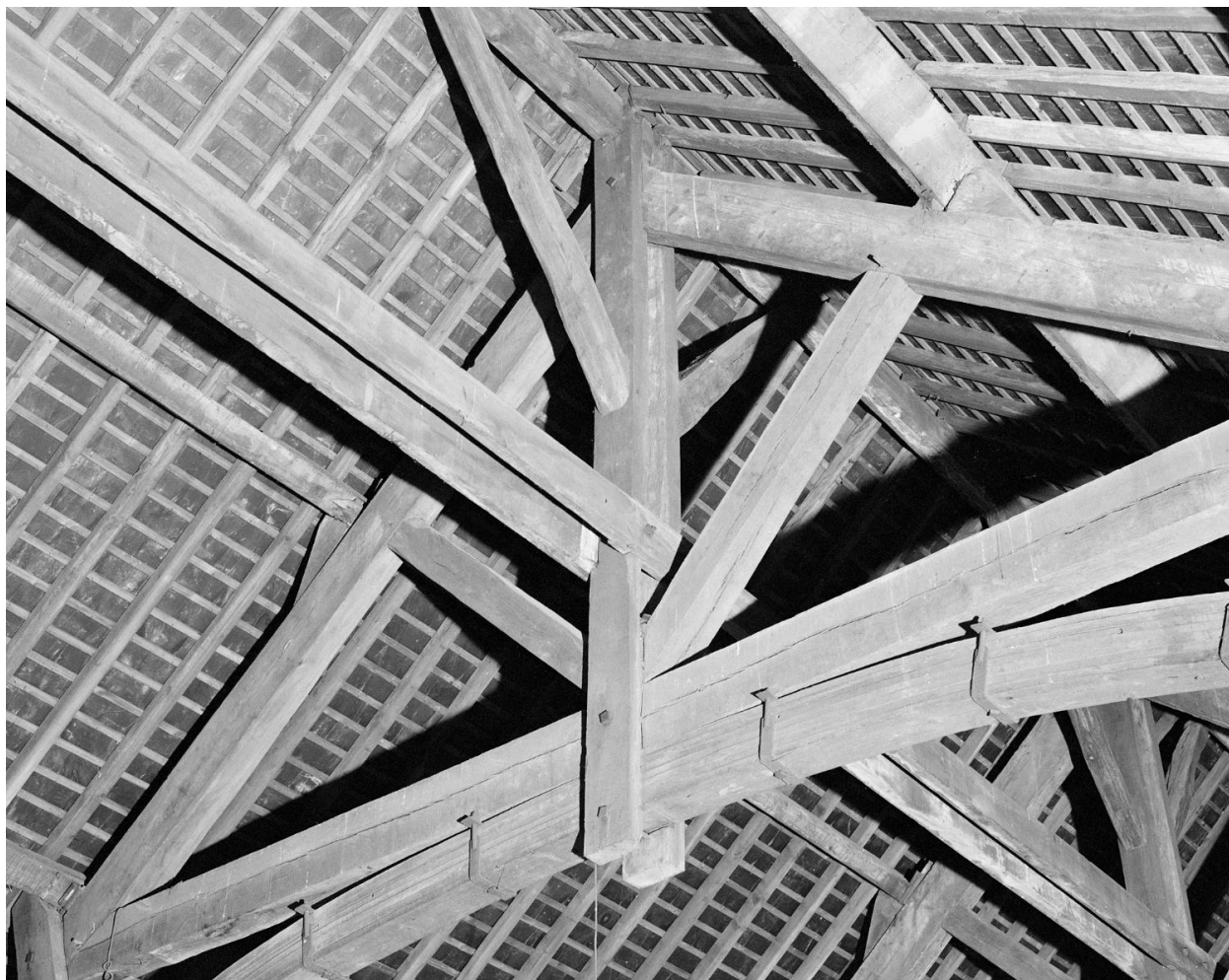
Charpente : vue sur entrait retroussé et double faîtage.
