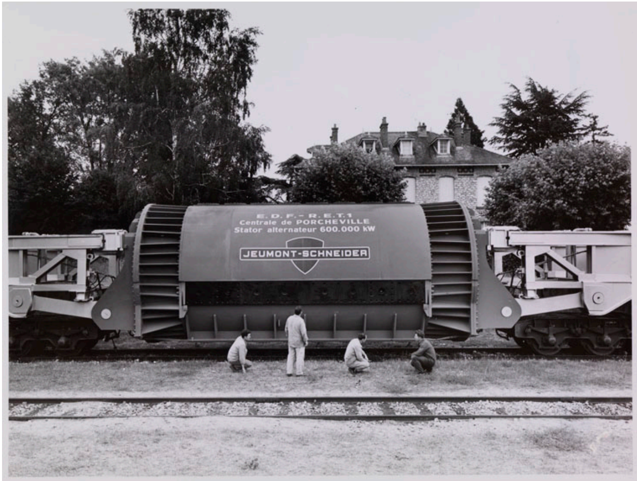
Photo ancienne. Turbo-alternateur 600MW pour la centrale EDF de Porcheville. Stator assemblé, posé sur un wagon spécial et prêt pour l'expédition. Photographie J-S, 17 juin 1967.
