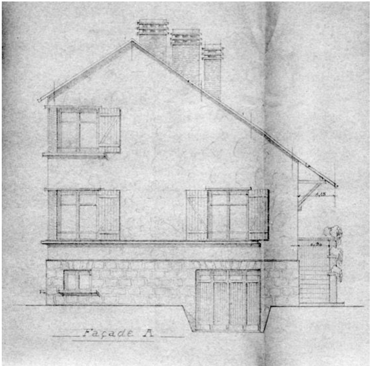
Projet de l'architecte melunais Louis Carrier pour une maison des "Castors de Melun nord" : la façade A. Tirage d'architecte, 1953. (AM Melun. 936 W 7)
