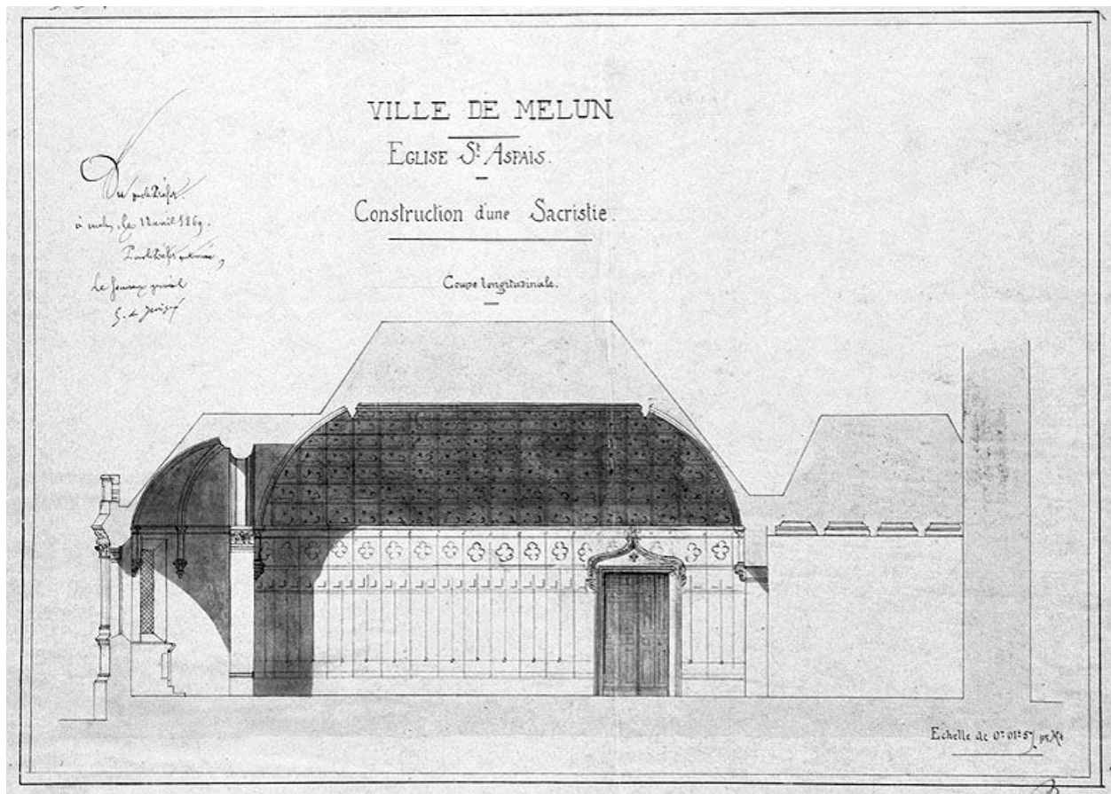
Ville de Melun. Eglise Saint-Aspais. Construction d'une sacristie. Coupe longitudinale. Echelle : 0.015 m.p.m. Calque aquarellé, 1869. (BM Melun. HH 28)
