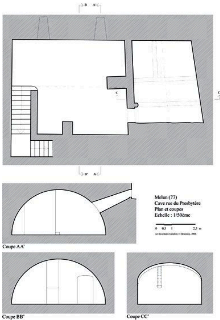
Plan et coupes de la cave.
