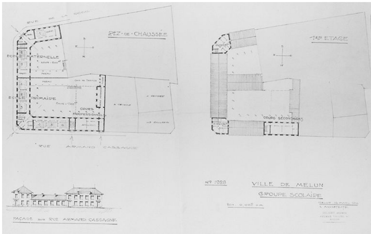
Plan au sol, plan du premier étage, façade sur la rue Armand Cassagne. Papier (tirage d'architecte), 16 mars 1910. (AM Melun. 1 Fi 727)
