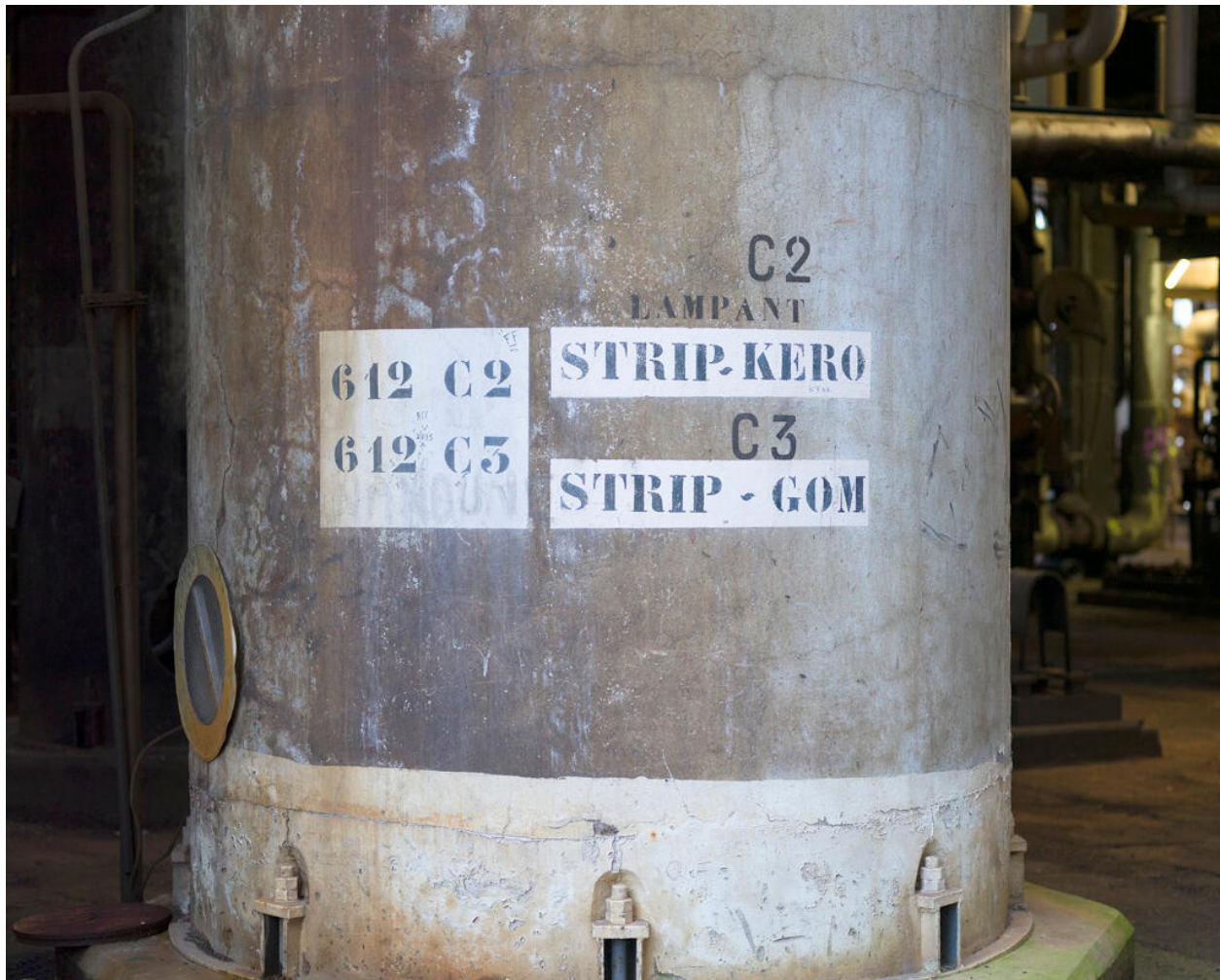
Unités Ouest - Zone de distillation (Unité 612). Marques de repérages des équipements ("lampant" étant l'ancien nom du kérosène).
