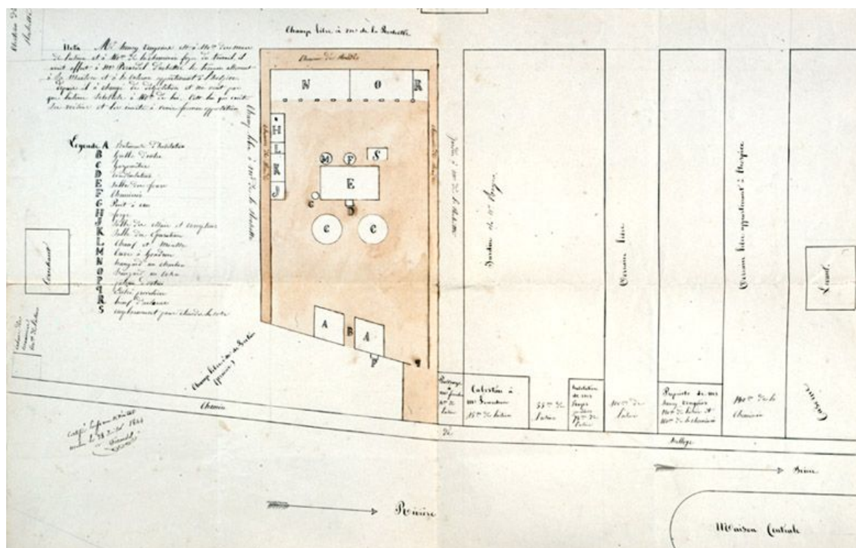
Projet de création d'une usine à gaz à Melun. Papier aquarellé, 18 juin 1844. (AD Seine-et-Marne. 5 Mp 303)
