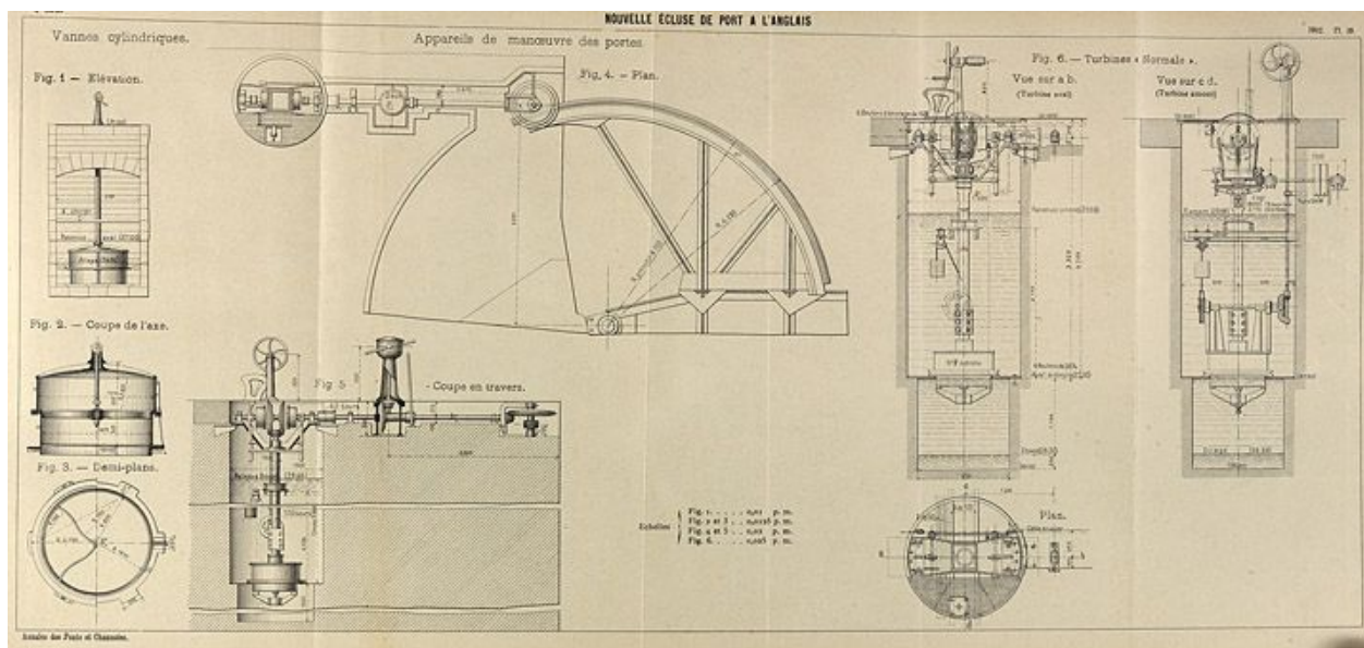
Alfortville, Vitry-sur-Seine. Barrage éclusé de Port-à-l'Anglais. Nouvelle écluse de Port-à-l'Anglais. Elévations, plans et coupes. Tiré de : Note sur la construction d'une nouvelle écluse à Port-à-l'Anglais sur la Haute-Seine / M. Alby. In Annales des Ponts et Chaussées, 3e trimestre 1902, n°30.
