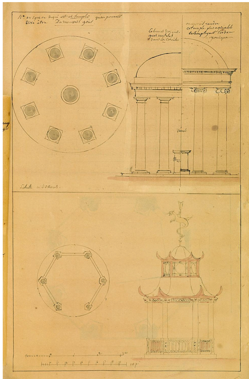
Relevé de fabriques du parc du château : le Temple de l'Amour et le Pavillon chinois, 1823. (Ecole nationale des ponts et chaussées, Champs-sur-Marne. Fonds Charles-François Mandar)
