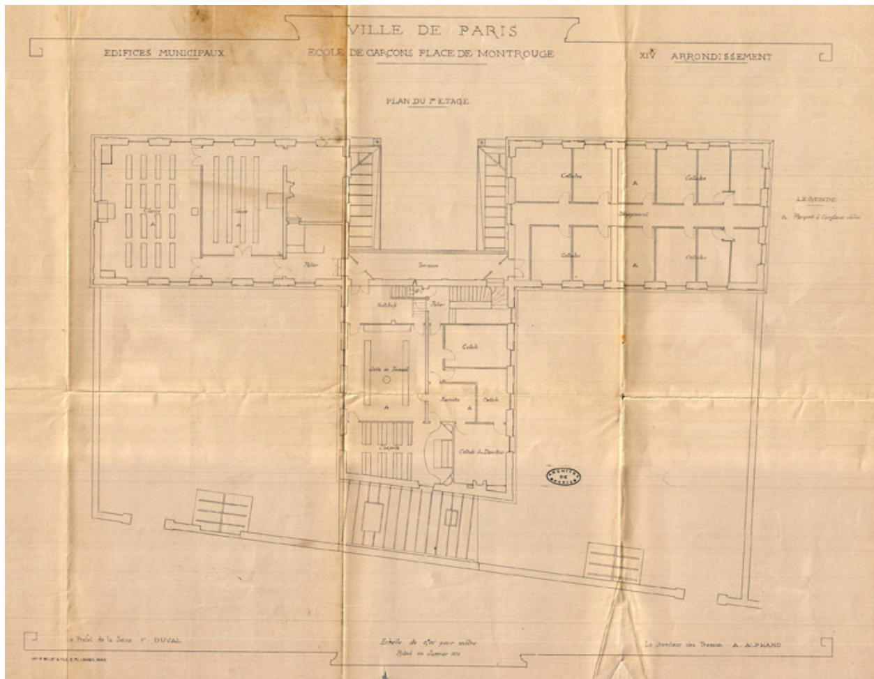
Plan du 1er étage de l'école de garçons, 1878. (AD75 V27 M4 art.1-13).
