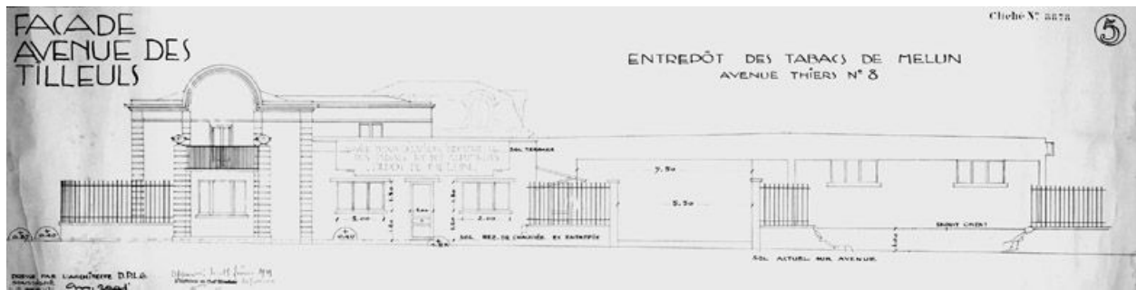
Entrepôt des tabacs de Melun : élévation sur l'avenue des Tilleuls (à l'angle de l'avenue Thiers). Tirage d'architecte, 1939. (AM Melun. 1 Fi 1448)
