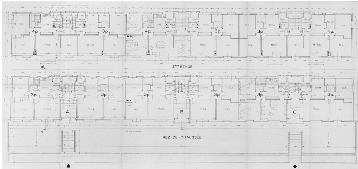
Plans des immeubles collectifs, rez-de-chaussée et 3e étage, par J. Thivier et R. Poggi, octobre 1955.
