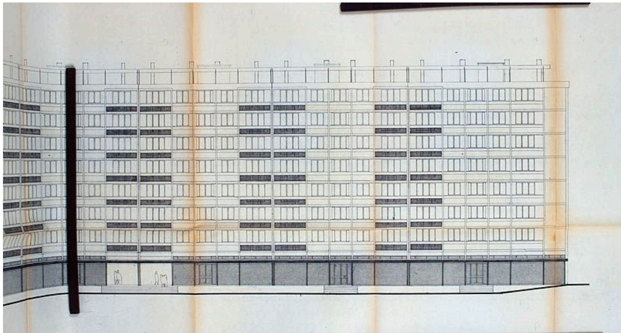
Cité dite Résidence Saint-Hubert. Plan de la façade avant d'un bâtiment donnant sur la place en U.
