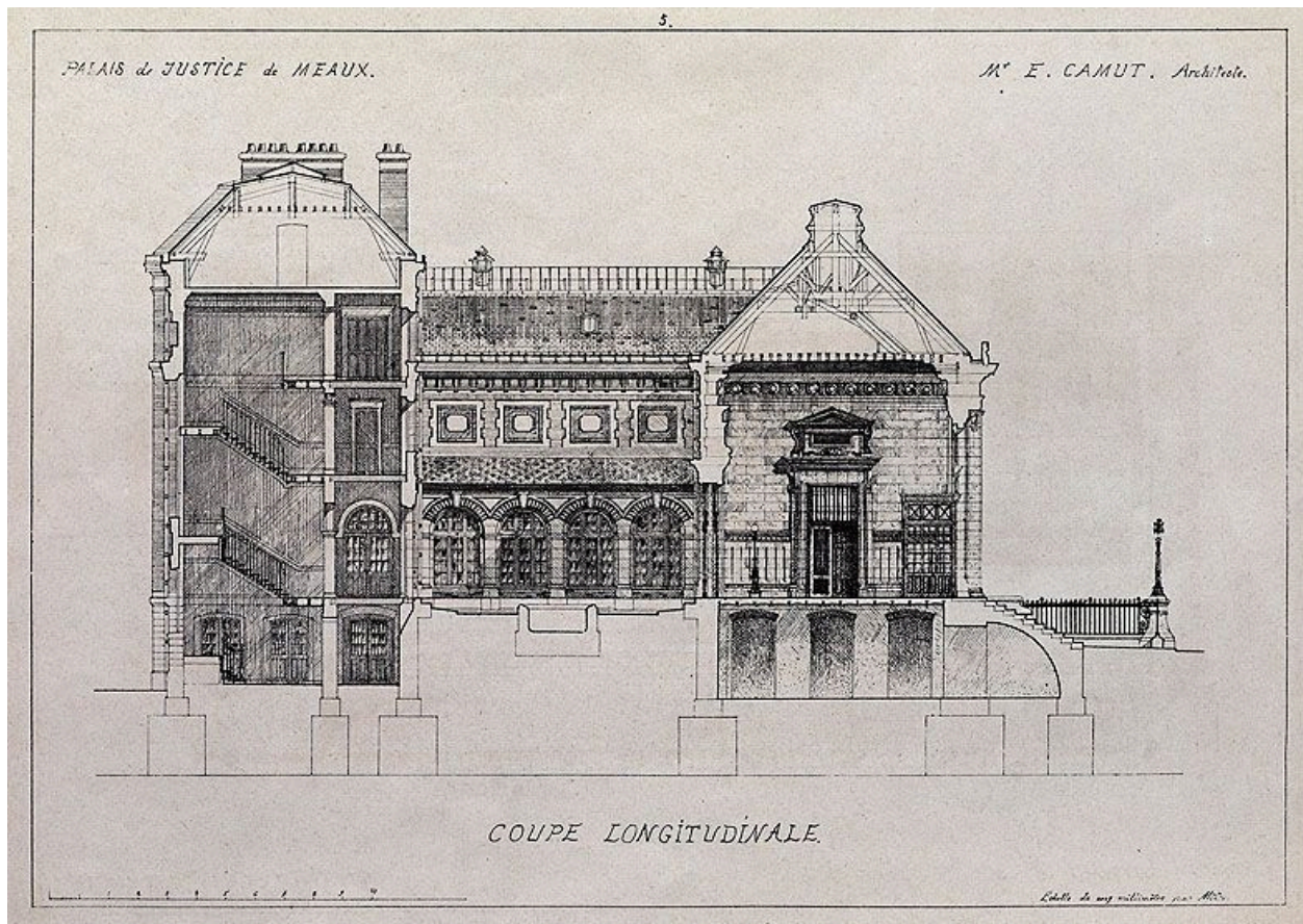
Le palais de justice de Meaux" : coupe longitudinale. Lithographie. Tiré de : "Monographies de bâtiments modernes" / A. Raguenet, p. 5. (Musée Bossuet, Meaux)
