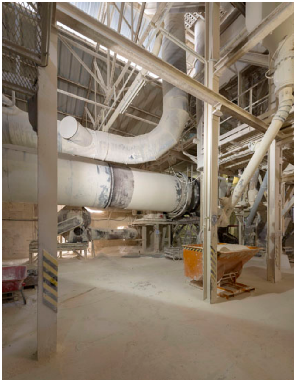
Usine de filler BR1. Séchage au gaz dans un cylindre rotatif VERNON (14x10m) avec filtre a manches.
