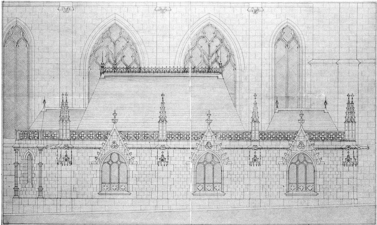
Ville de Melun. Eglise Saint-Aspais. Sacristie nouvelle, projet définitif. éch. 0.03 m.p.m. Calque aquarellé, 12 juin 1868. (BM Melun. HH 24)
