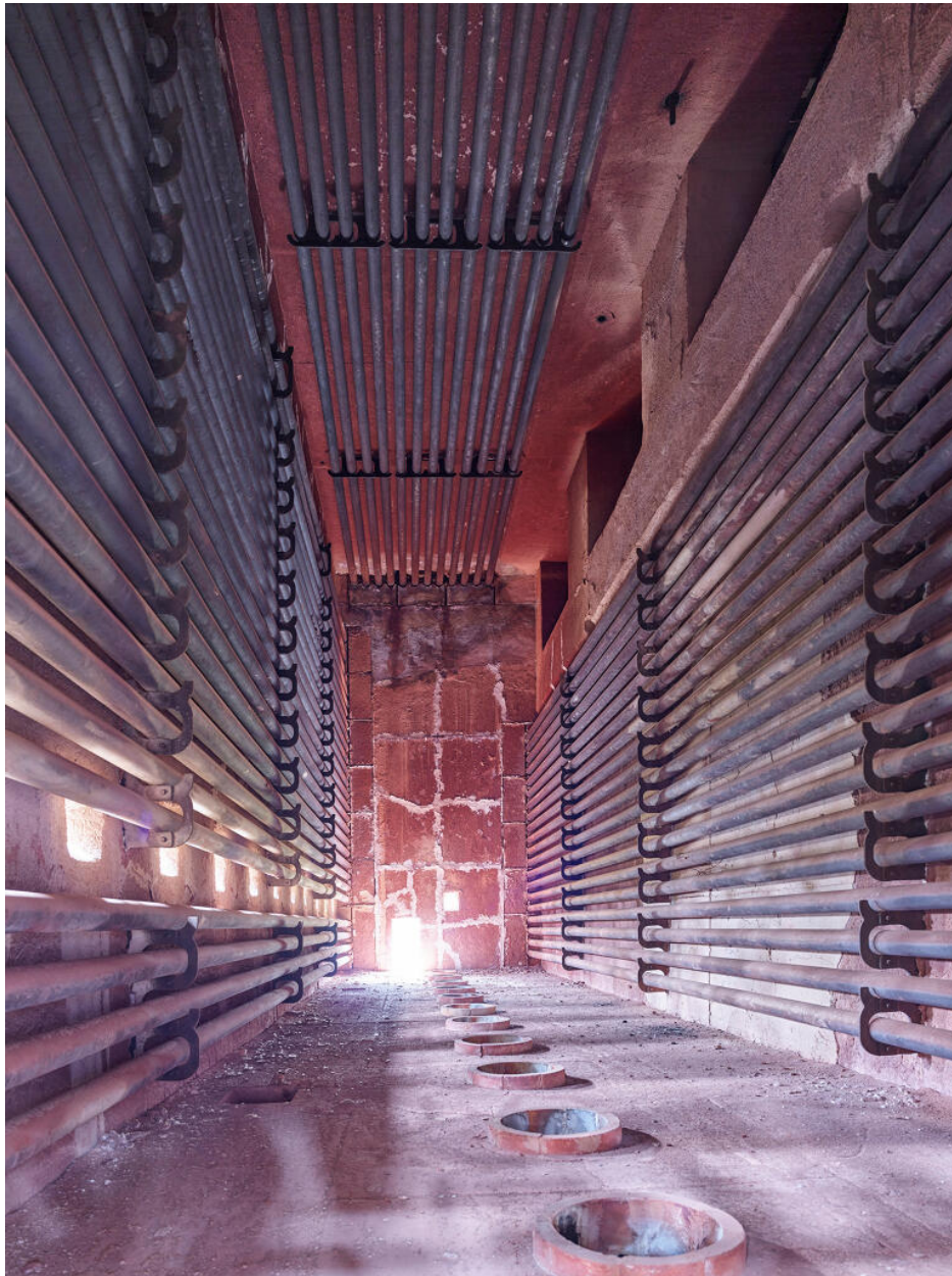
Unités Est - Zone du viscoréducteur (Unité 691). Vue intérieure du four de l'unité. Le produit à réchauffer circule dans les tubes, les brûleurs sont en bas.
