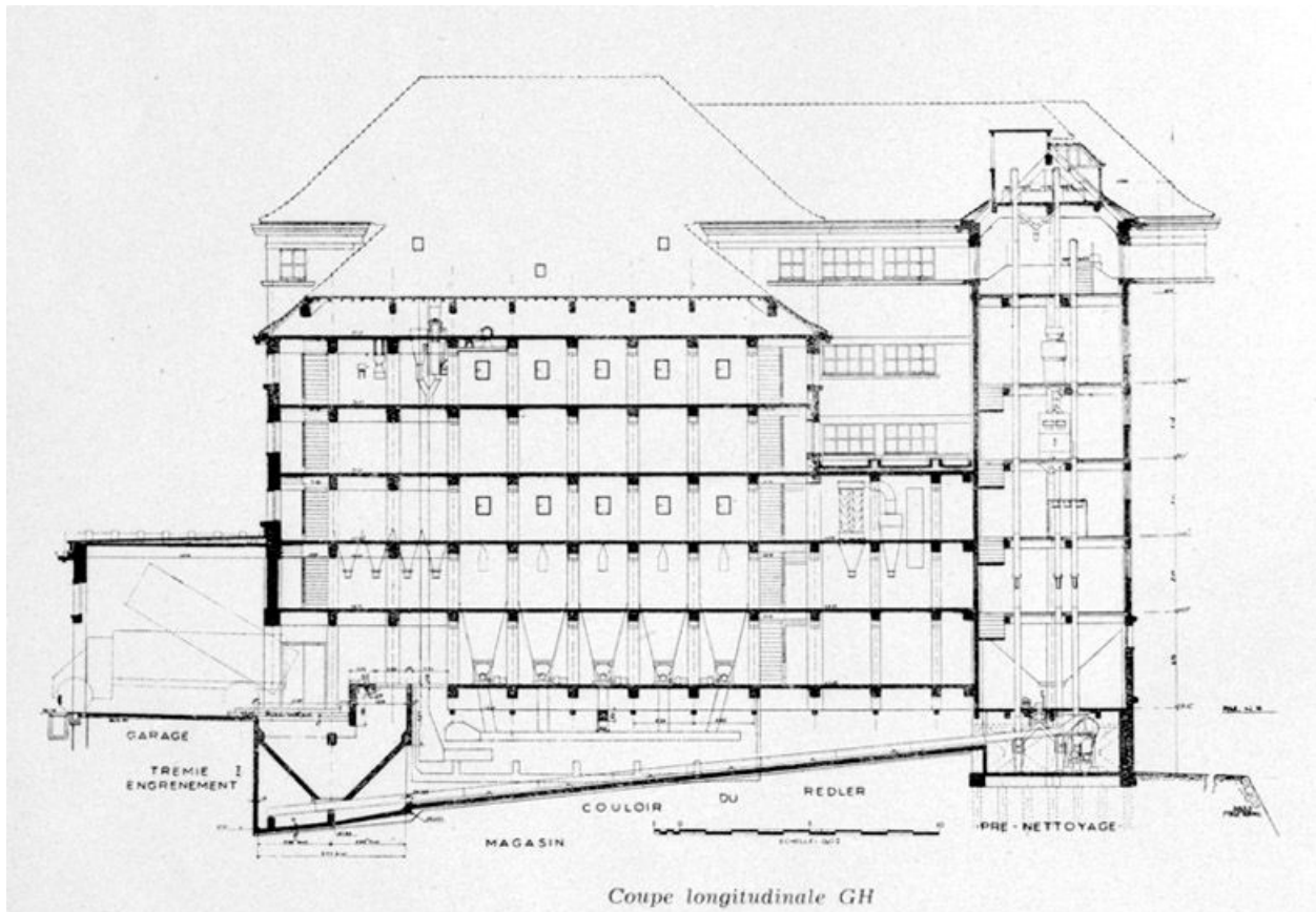
Coupe longitudinale GH. Photogravure, 1949. Tiré de : L'Architecture française, constructions industrielles (II), n° 85-86, 1949. (AM Melun. 578 W 3)
