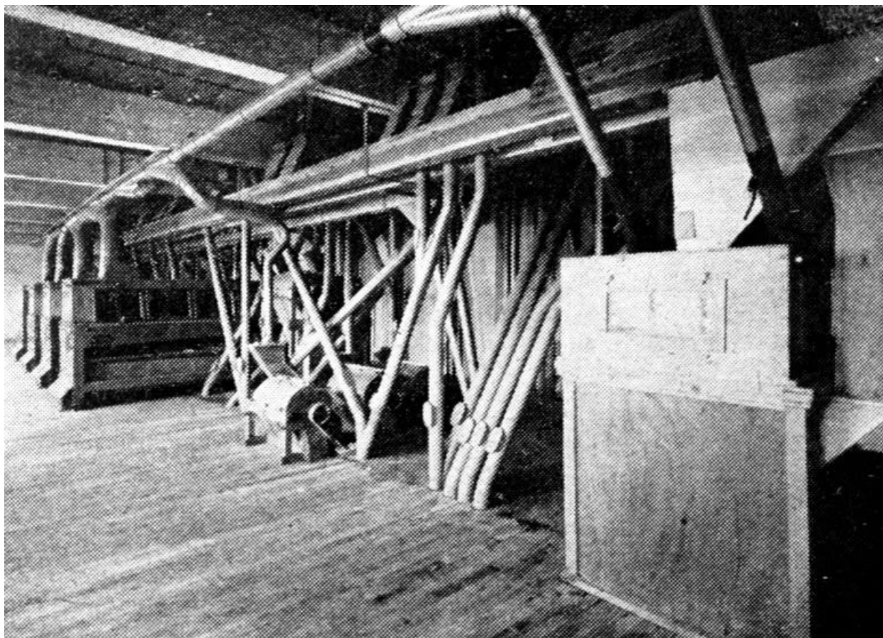
Sasseurs et conduits métalliques, au troisième étage de la minoterie. Tiré de : Les nouveaux Moulins de Melun, dans La Meunerie française, n° 27, septembre 1948. (Conservatoire national des arts et métiers. Pt Fol Ku 17)
