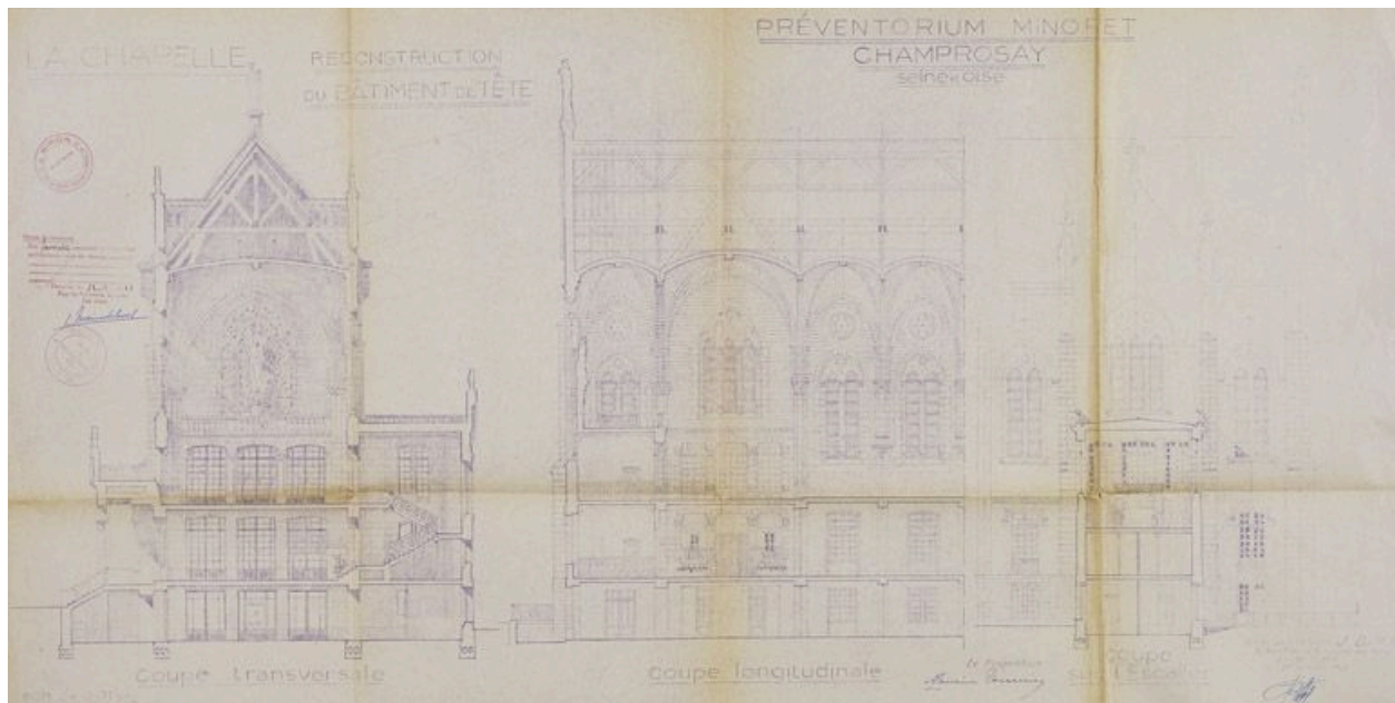
Plans pour la reconstruction de la partie antérieure de la chapelle détruite par le bombardement aérien du 29 mai 1944 : coupes transversale, longitudinale et sur l'escalier. (AD Essonne, 902 W 21)
