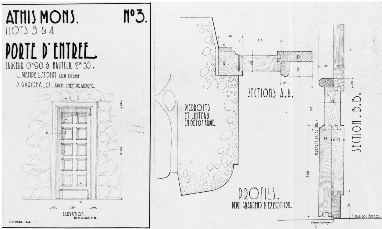
Ilots 3 et 4 : élévation et profil des portes d'entrée ; L. Mendelssohn architecte en chef, P. Garofalo architecte chef de groupe, octobre 1948.
