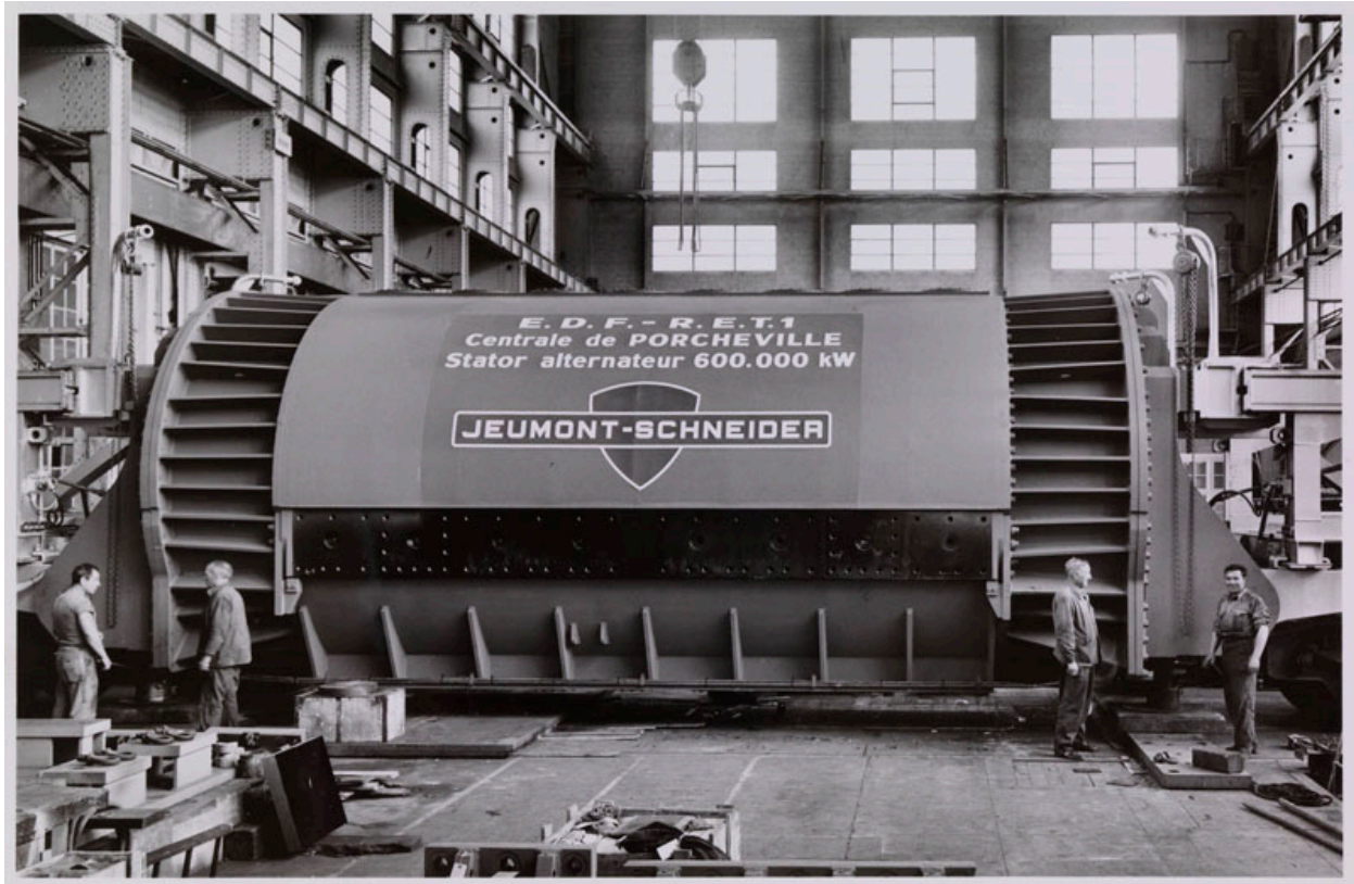
Photo ancienne. Turbo-alternateur 600MW pour la centrale EDF de Porcheville. Stator assemblé, posé sur un wagon spécial et prêt pour l'expédition. Photographie J-S, 17 juin 1967.
