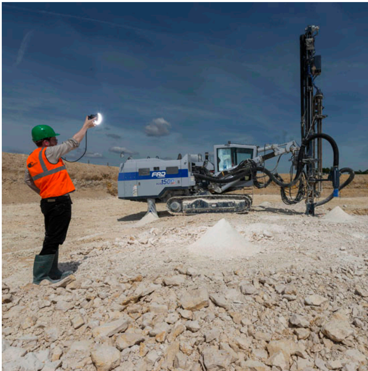
Front de carrière. Formation calcaire de Champigny et de Chateau-Landeu. Dépôt lacustre.
