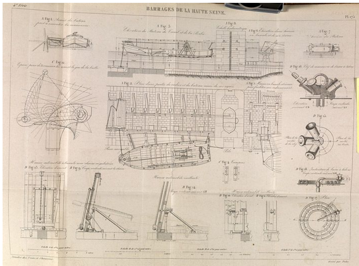
Barrages de la Haute-Seine. Bateau de manoeuvre des hausses. Elévations et coupes. Tiré de : Mémoire sur la construction des douze barrages éclusés, exécutés sur la haute Seine entre Paris et Montereau / M. Chanoine et M. de Lagrené. In Annales des Ponts et Chaussées, 2e semestre, 1868, n° 200, pl. 174-175.
