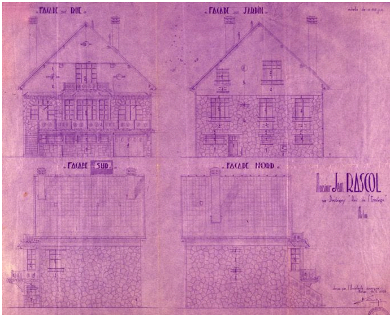
Pavillon de M. Jean Rascol rue Daubigny. Papier, tirage d'architecte, 1939. (AM Melun. 1 Fi 1450)
