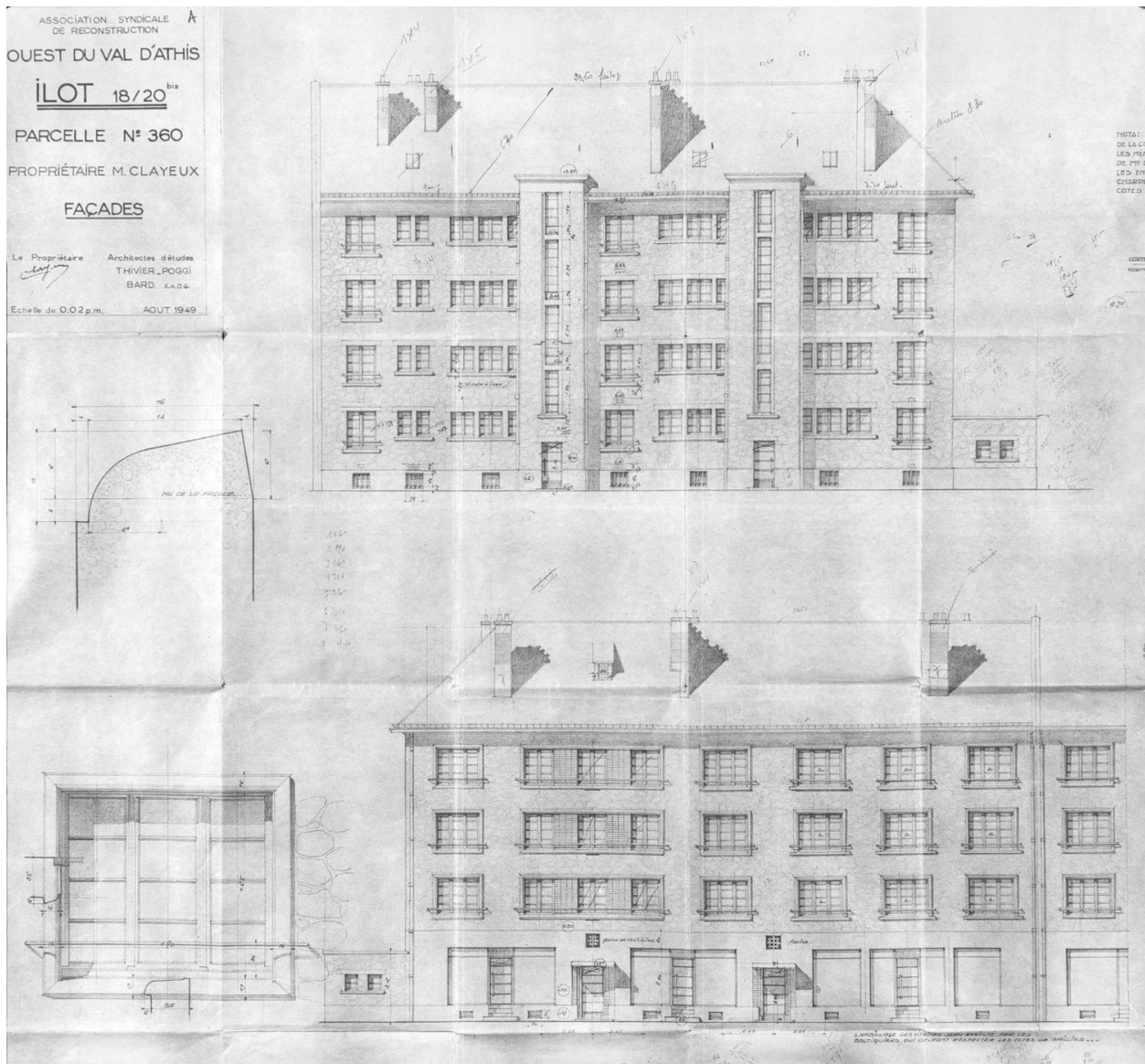
Elévations et détail de fenêtre de l'immeuble Clayeux (mitoyen avec l'immeuble Dervaux) situé 4-4bis, place Jean-Jaurès ; Thivier, Poggi et Bard, architectes d'études ; 9 août 1949.
