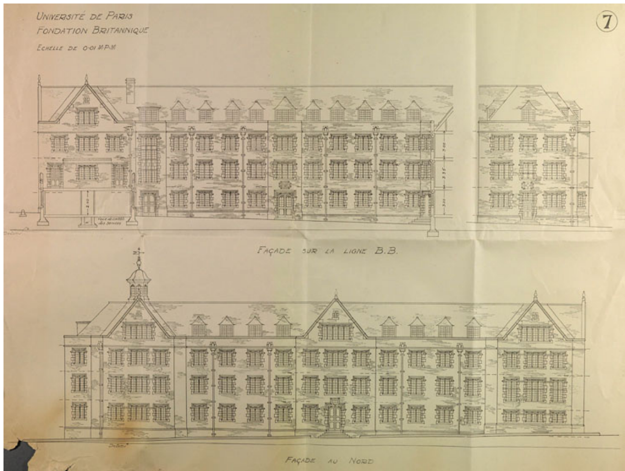
Façade nord, s. n., s.d. [Pierre Martin et Maurice Vieu, 1931]. Plan. Archives nationales, AJ 16/7041.
