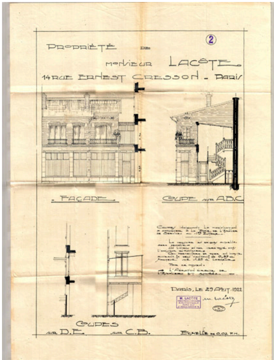
Façade immeuble sur cour, propriété de Monsieur Lacôte. -Plan, 1922. (Archives de Paris, VO11 1131).
